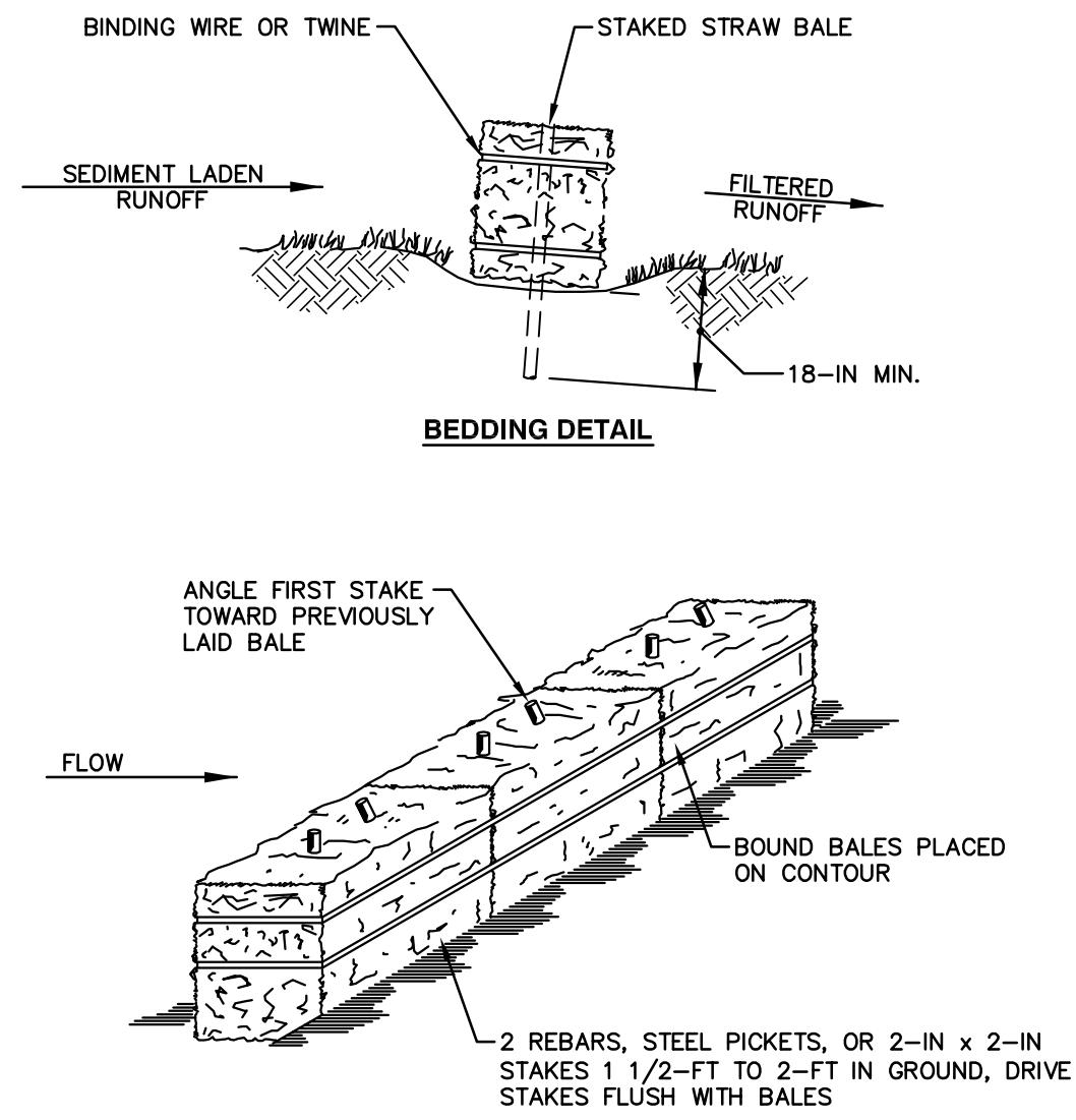
DETAIL D HAY BALES N.T.S.
